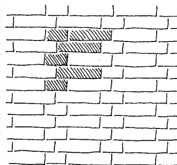
Munke forbandt
