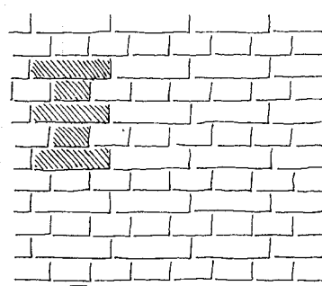
Blokforbandt
