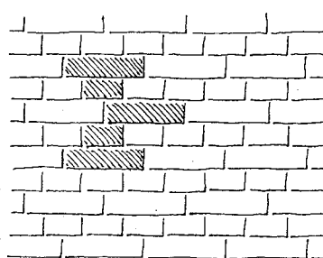
Krydsforbandt
